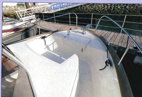
Une banquette biplace est placée devant la timonerie. L'accastillage comprend un davier, des chaumards et des taquets. Des coffres sont accessibles sous le plancher du cockpit.
