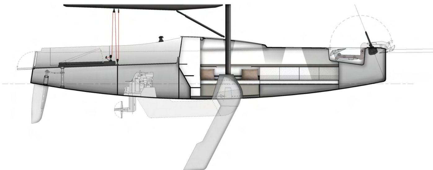
Plan d'aménagement principal - 2
