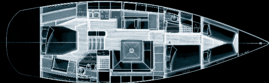
Version cabine avant latérale / Forward starboard cabin
