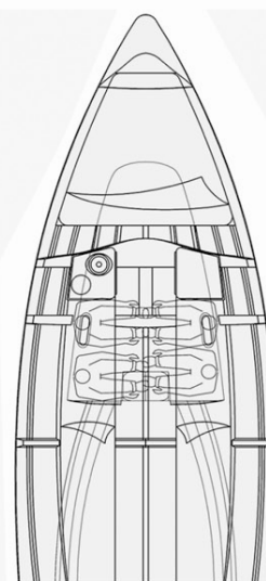
Plan d'aménagement Version croisière
